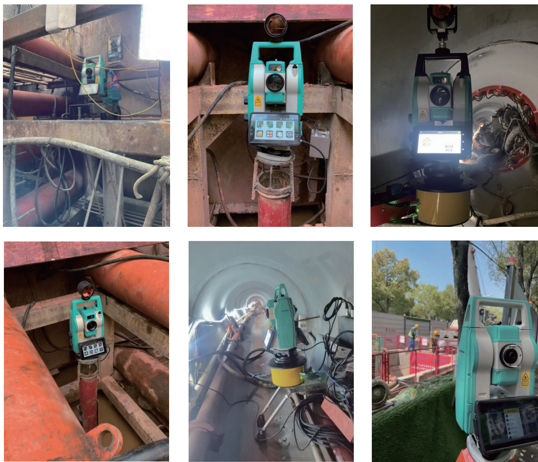
「湖南长沙顶管现场图」
